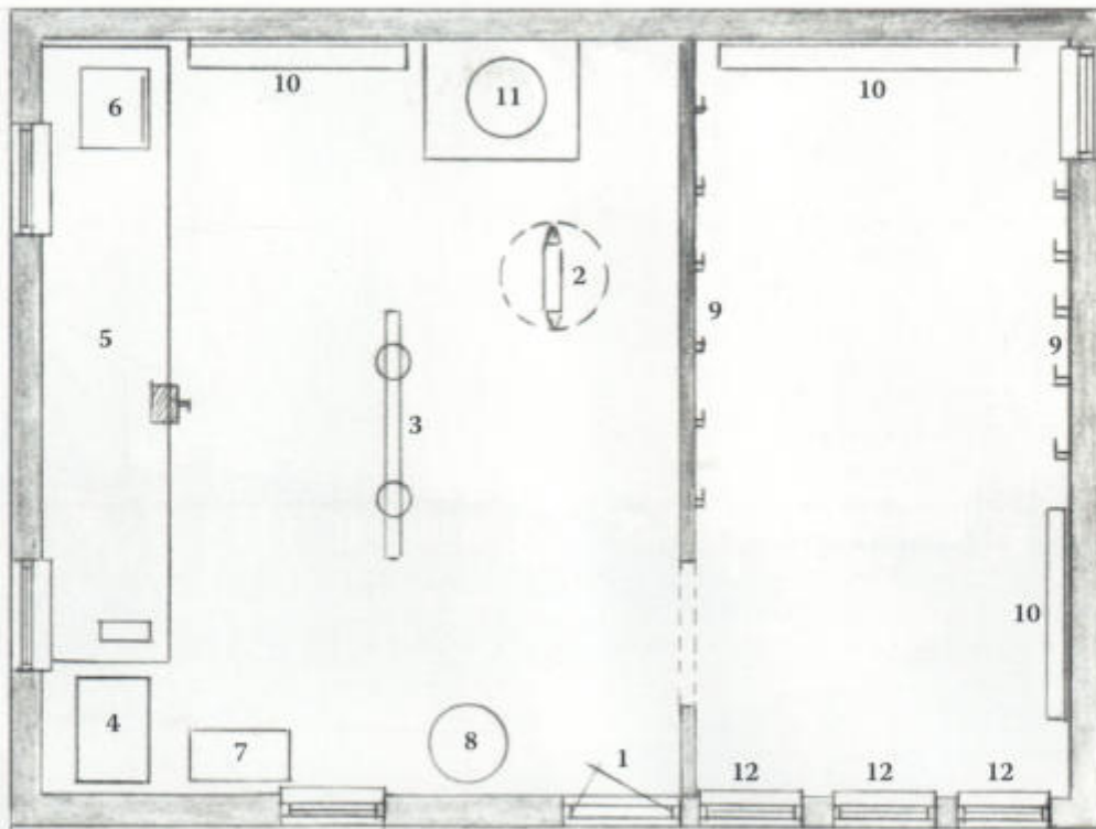
Plattegrond van de werkplaats van fietsmaker Hendrik Geene te Maren. Een keet van 6 x 8 meter die vlak na de oorlog nog dienst had gedaan als noodwoning, werd in 1948 gedemonteerd en opnieuw opgebouwd achter het huis van de fietsmaker: 1. Toegangsdeur 2. Aambeeld 3. Ophanging voor reparatie en de zelfgemaakte waterbak op pootjes om gaatjes op te sporen 4. Slijpsteen 5. De werkbank met de bankschroef en een vaste boor links 6. Lessenaar voor administratie 7. Benzineopslag 8. Boormachine 9. Haken voor fietsbanden 10. Kasten en rekken voor opslag 11. Smidsvuur 12. Etalage.
